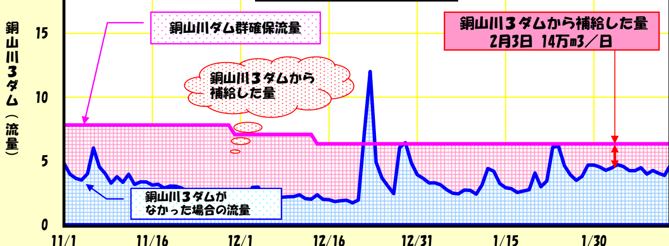
銅山川3ダム合計の流況
