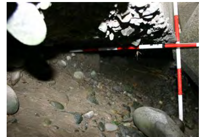
台風14号 吉原箇所 洗掘状況
