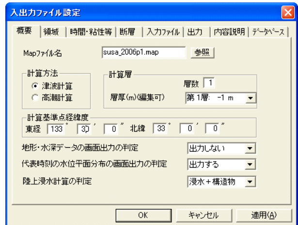
図-5 津波数値計算ソフトウェアシステムの画面例
