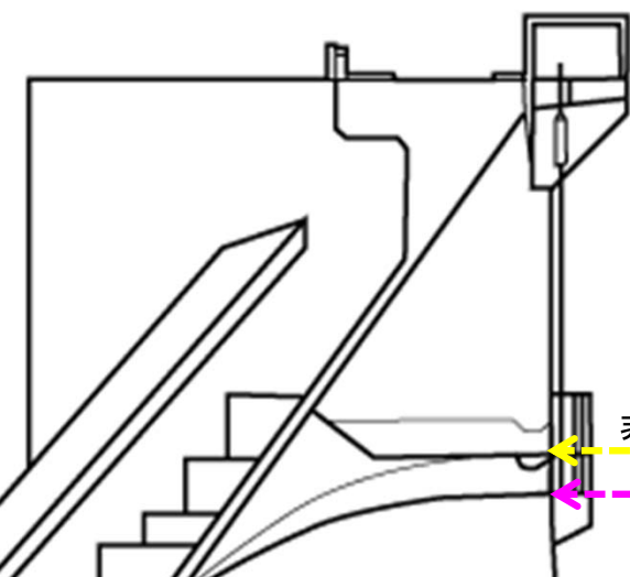
中筋川ダム断面図
