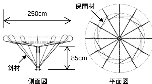
図-4 人工巣台「SS-3型」
