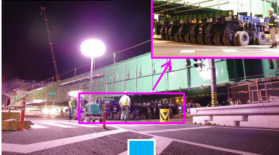
多軸式特殊台車による 橋桁運搬
