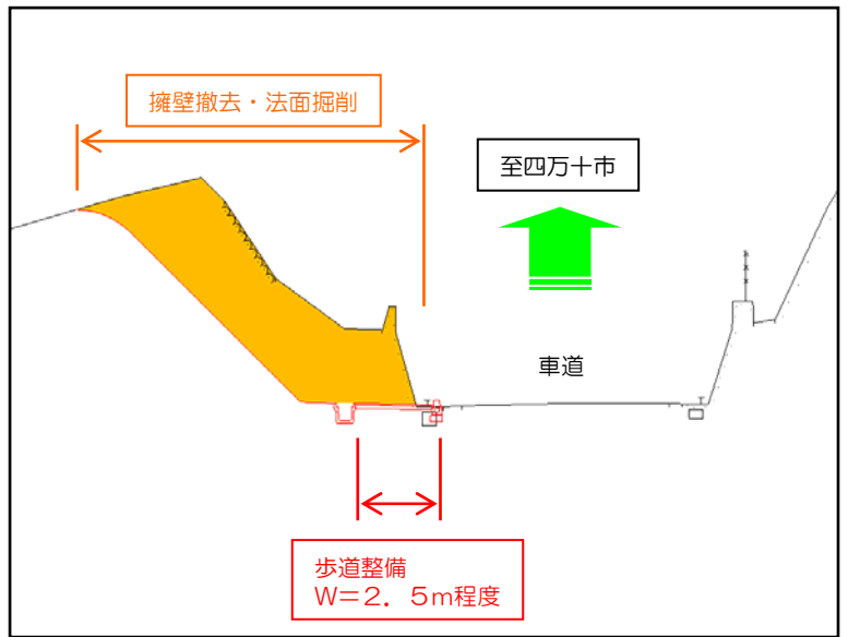
【横断面図】
