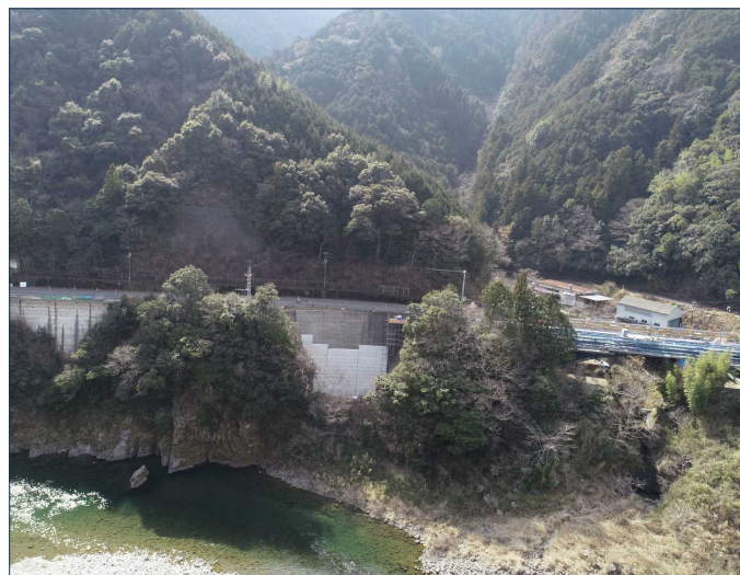
終点側工区（撮影方向：南西向き）
