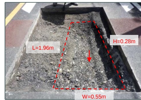
開削状況
