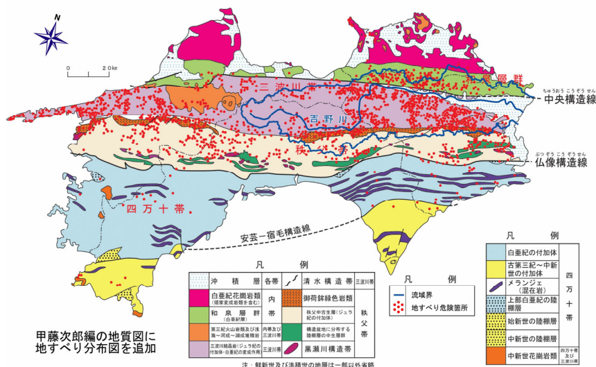
図－1.1.4 吉野川流域の地質
