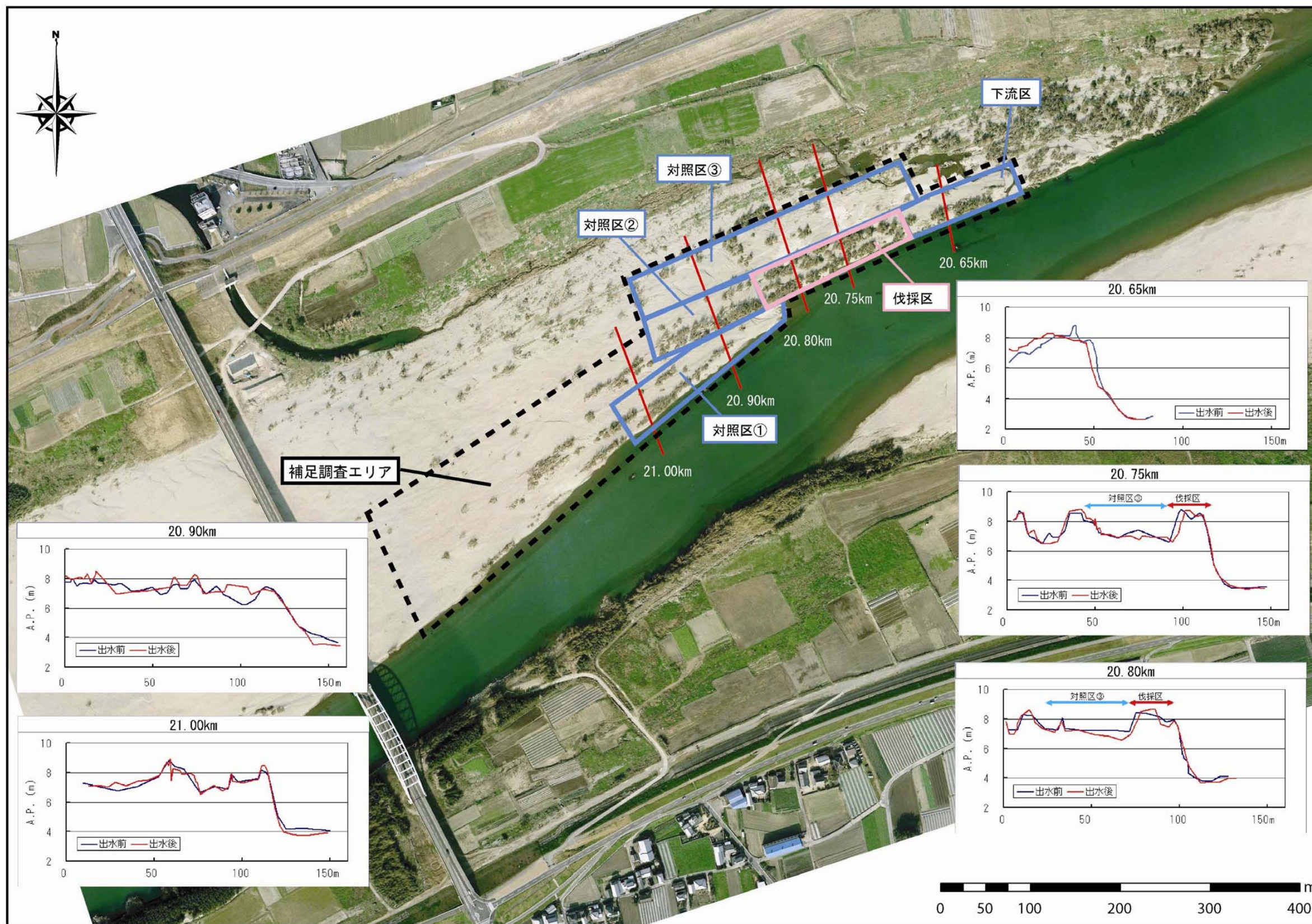
図 4.9 ヤナギ伐採区及び対照区における出水前後の横断方向の地形（標高）変化
