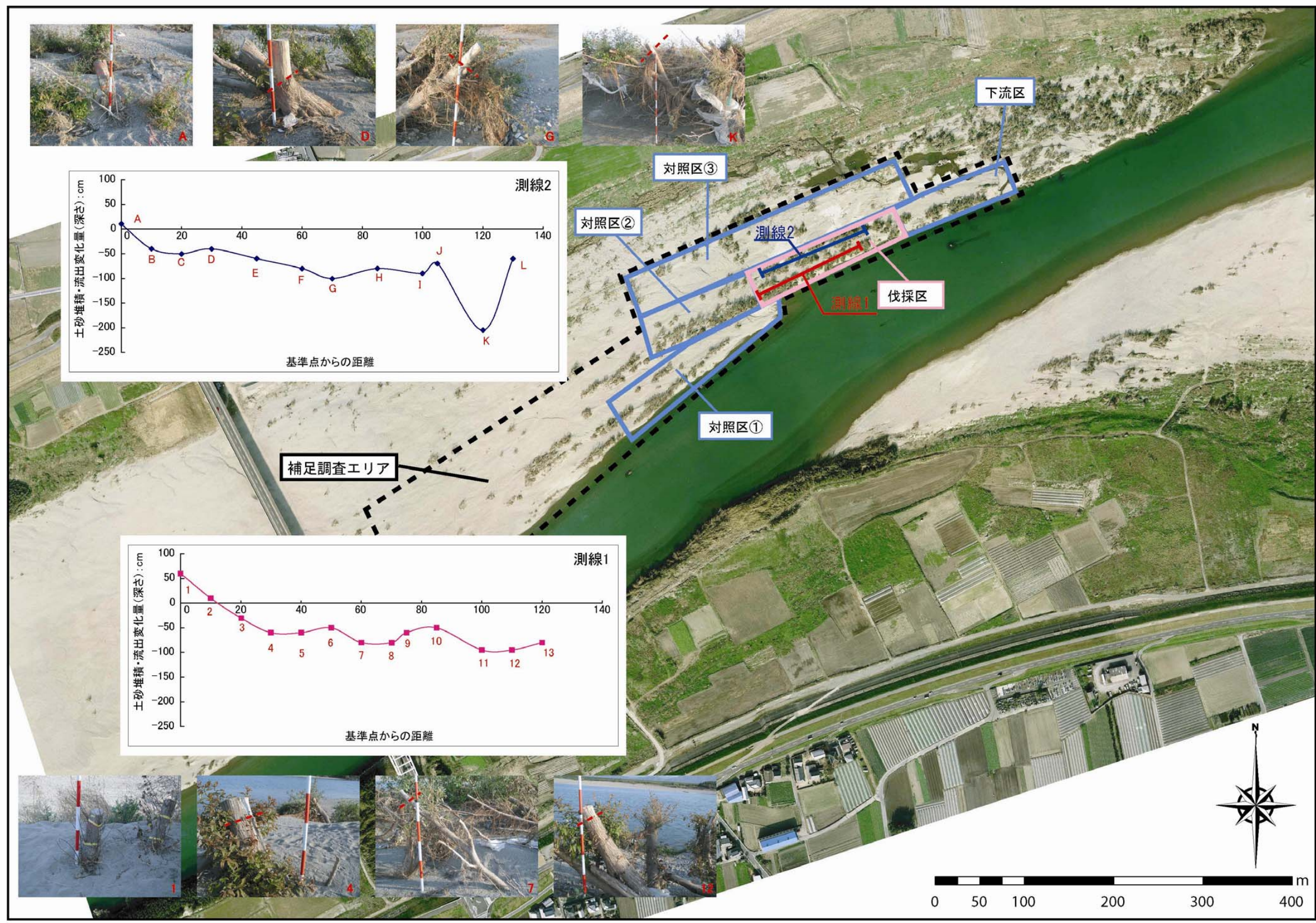
図 4.10 ヤナギ伐採区及び对照区における出水前後の縦断方向の地形（標高）変化
