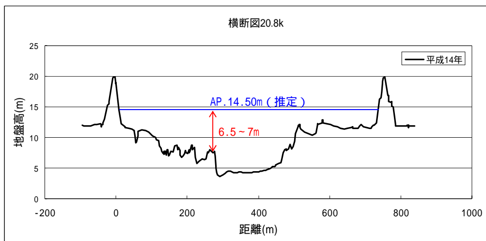
図 4.6 20.80km 地点の冠水位（推定）
