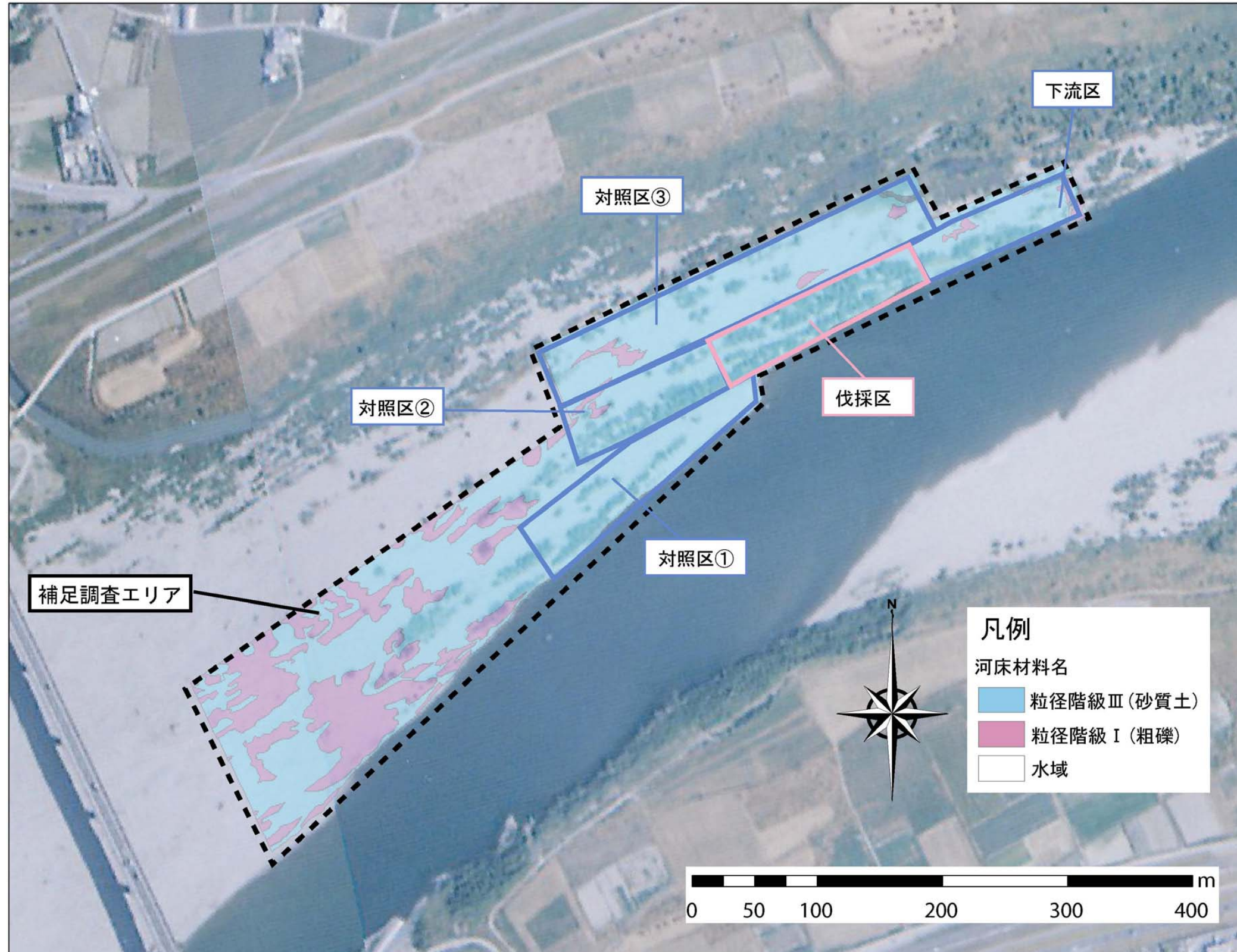
図 4.8 出水前の河床材料分布図（平成 17 年 8 月 25・26 日）
