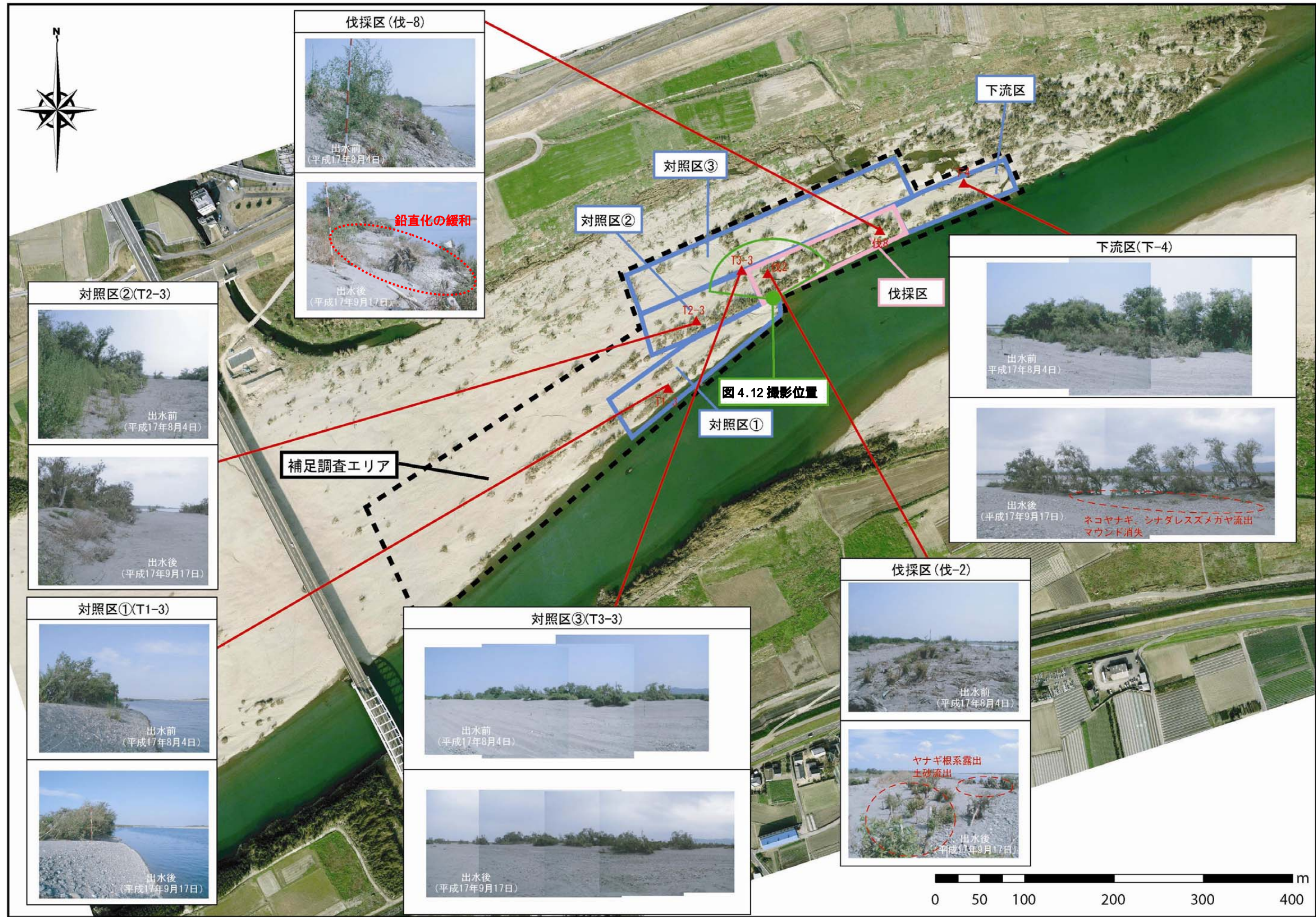
図 4.11 出水による地形及び河床材料の変化の概況
