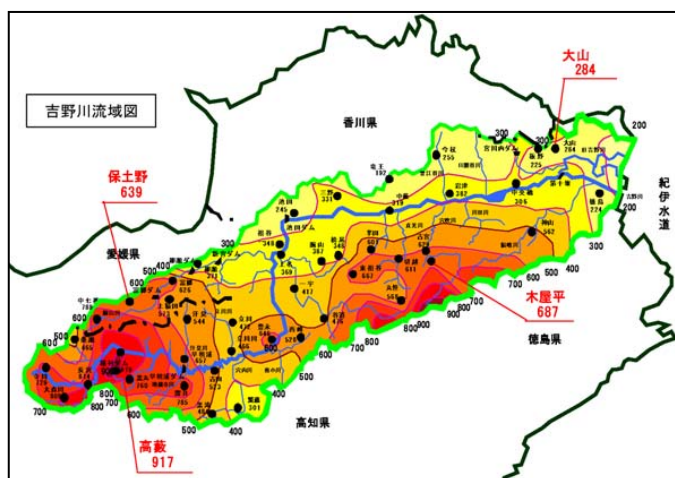
図 4.4 吉野川流域の等雨量線図（9 月 4 日～6 日） 出典：徳島河川国道事務所 HP より
