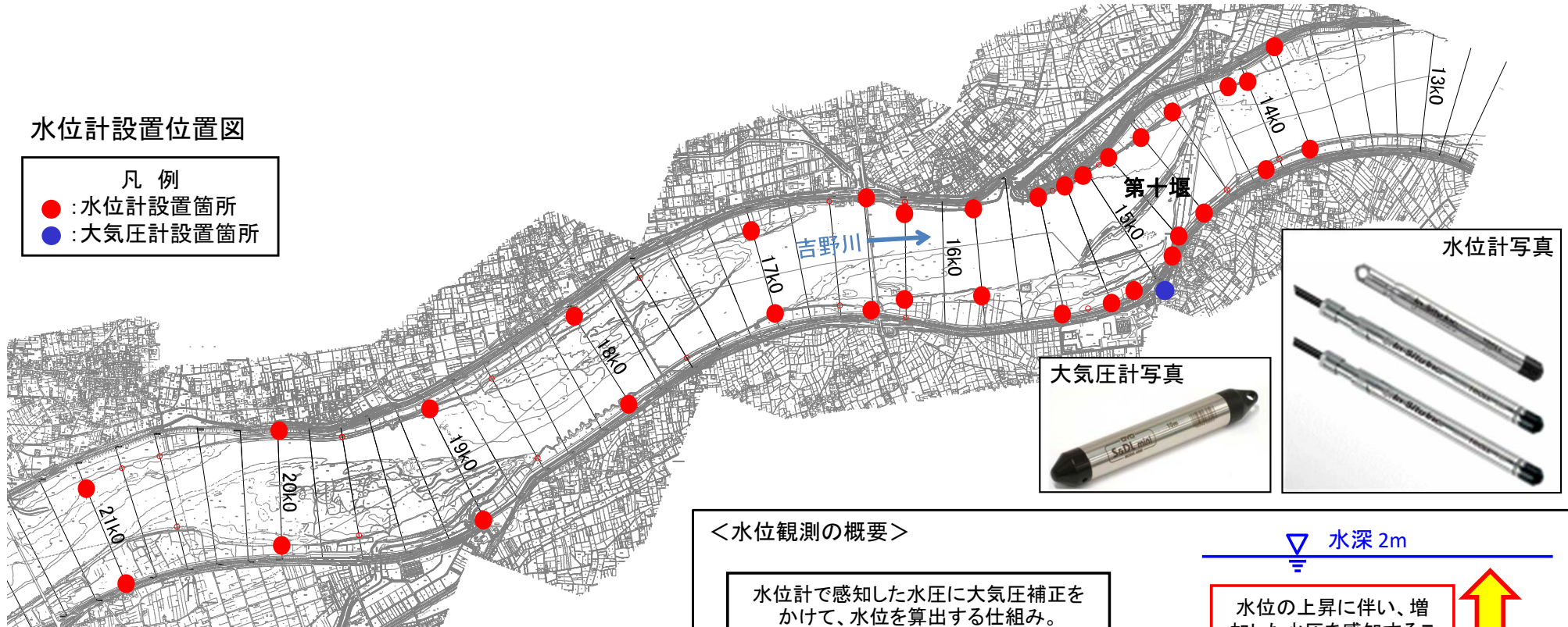
水位計設置状況
