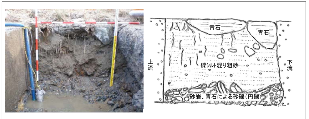
掘削側面スケッチ図
