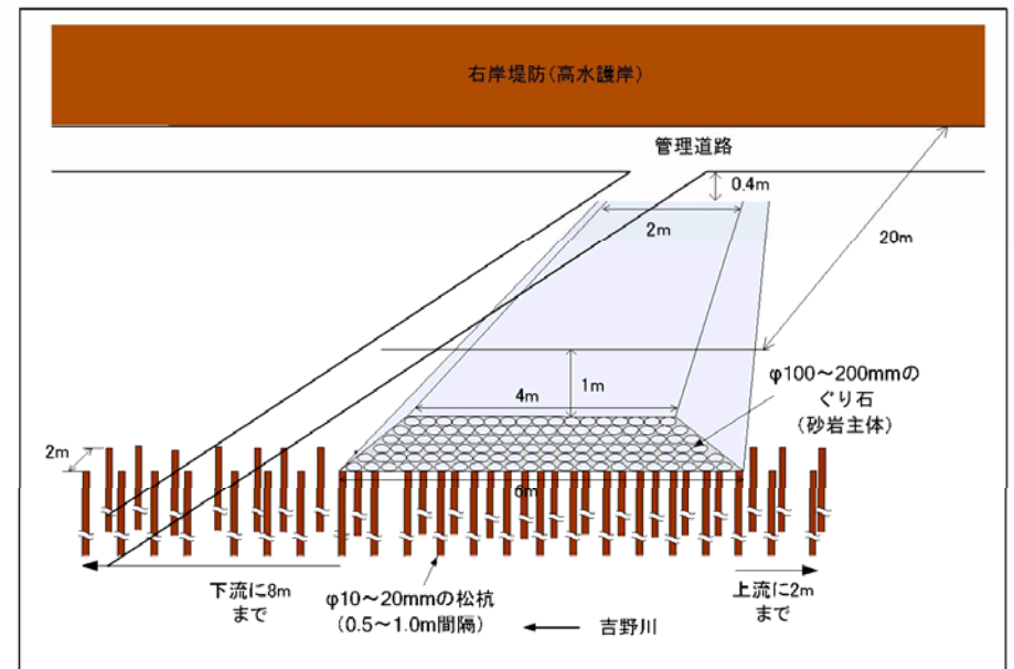
上堰-堰取付部付近の模式図
