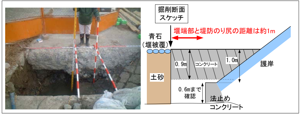
開削調査結果
