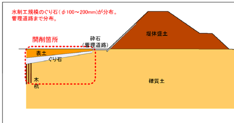
上堰-堰取付部構造調査結果
