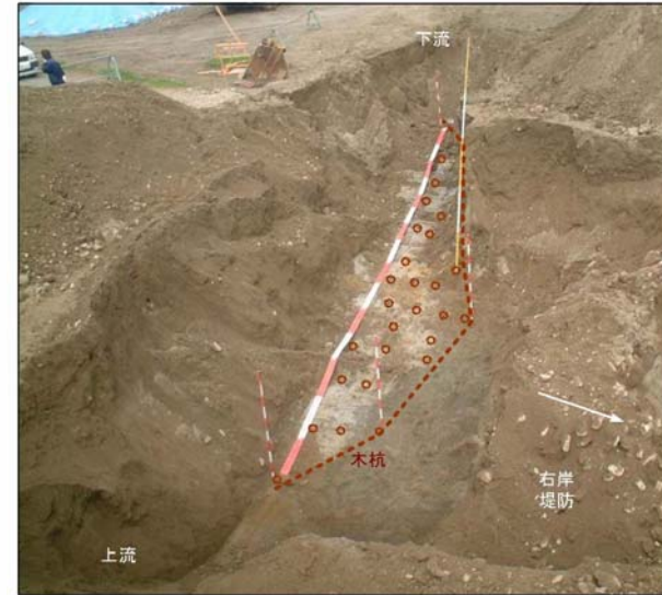
開削写真 (木杭の分布範囲)
