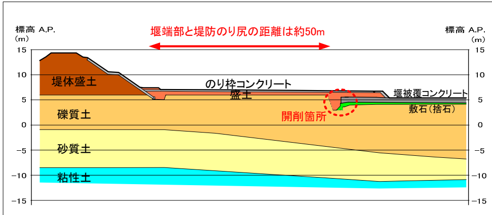
断面模式図
