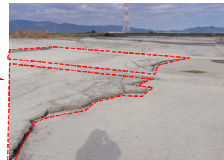
仮設道路(中詰めコンクリート)
