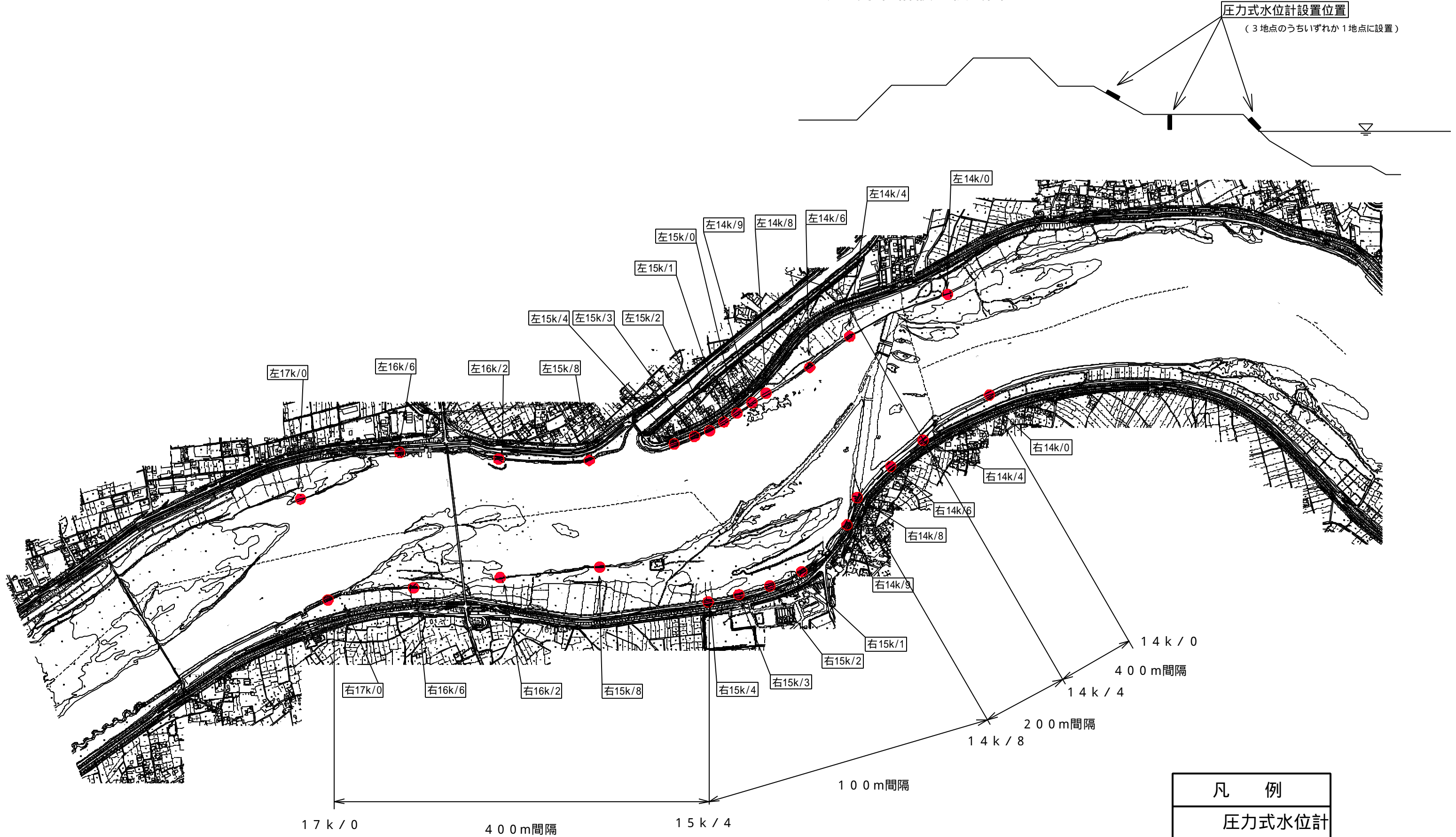
圧力式水位計設置模式図
