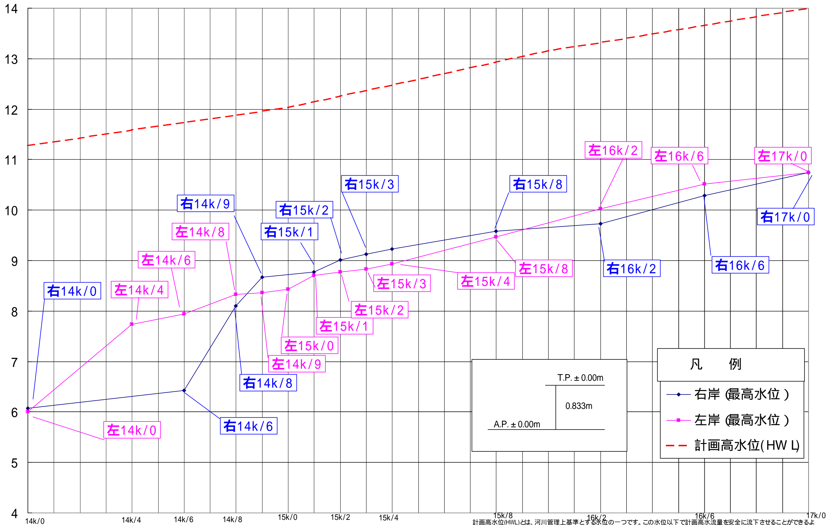
第十堰周辺の圧力式水位計による水位観測縦断図 (平成 16年 9月 30日 台風 21号)
