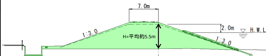
堤防の断面図 A-A
