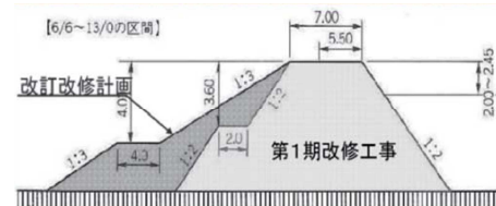
図-2 第二期改修事業の堤防補強のイメージ
