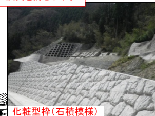
護岸工により洪水時の地山の浸食を防ぎます。
