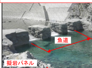
床固工により河床の安定を図ります。
