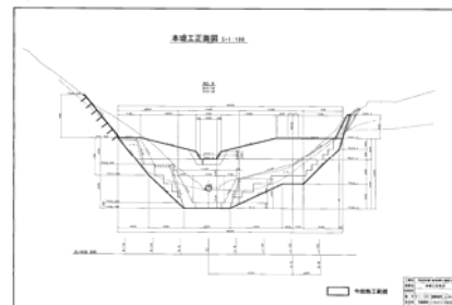
計画正面図
