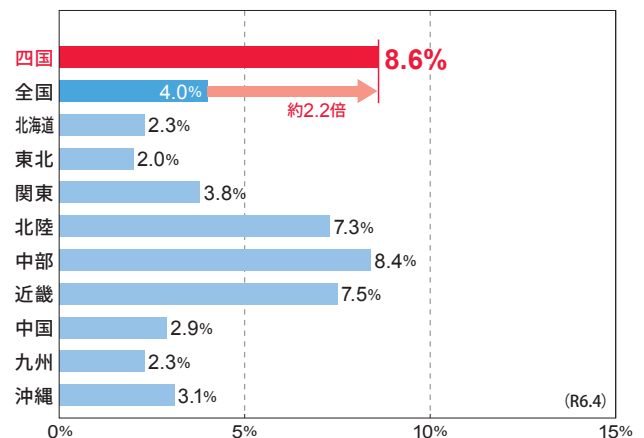
■直轄国道における事前通行規制区間率
