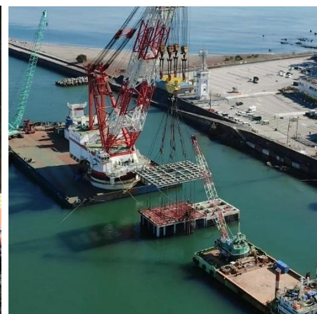
高知港海岸直轄海岸保全施設整備事業(高知県)
