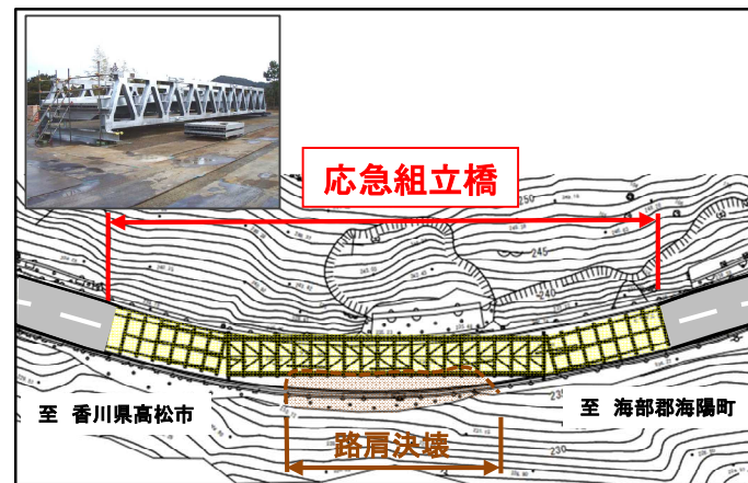
▲応急復旧工法 (応急組立橋活用)
