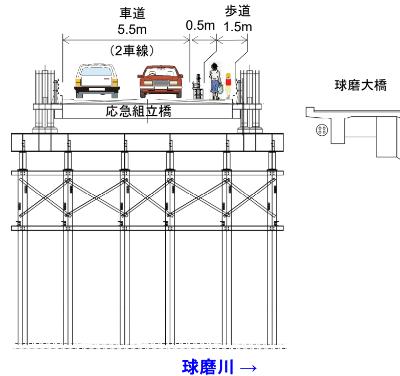
応急組立橋断面図
