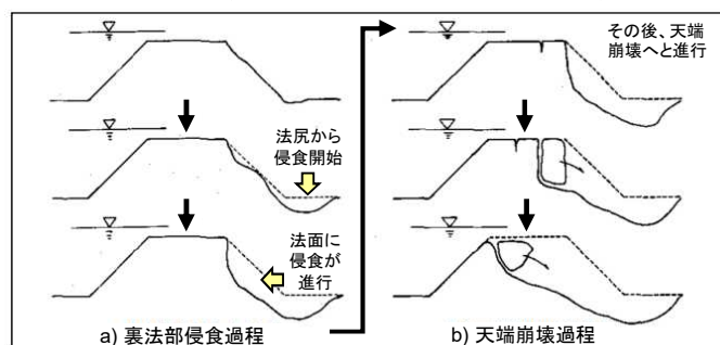
図-4 越水による河川堤防の壊れ方
