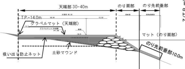
土砂流出防止工（標準断面図）
