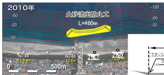
土砂流出防止工（平面配置）
