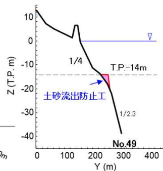
土砂流出防止工（断面図）
