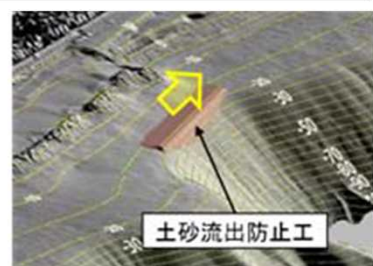
土砂流出防止工（海底鳥瞰図）
