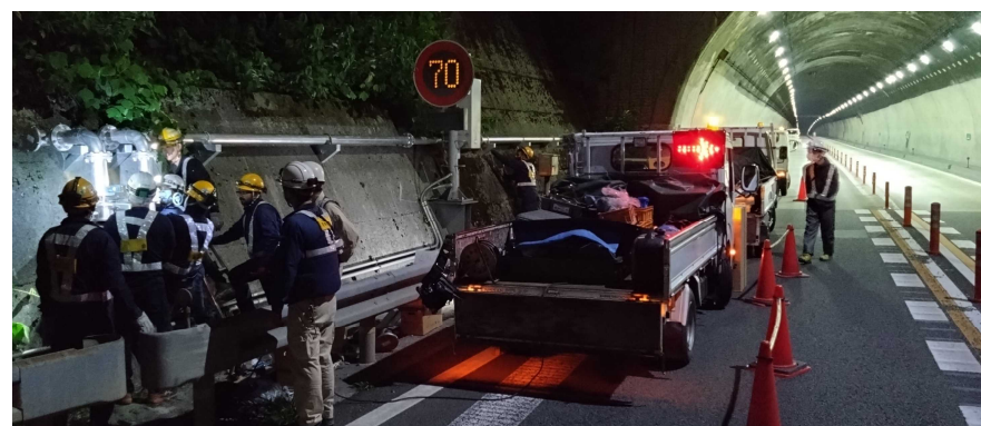
トンネル非常用設備設置作業
