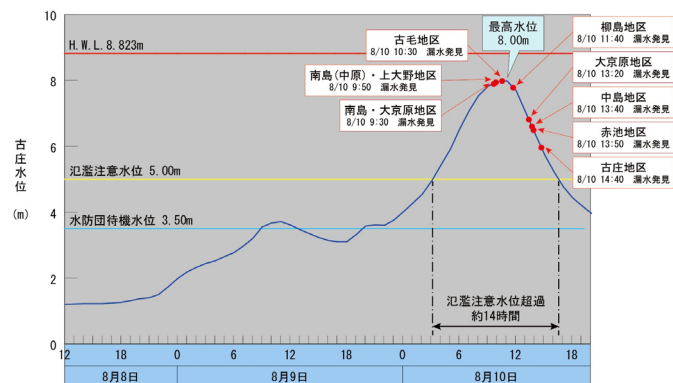
図-2.1.22 平成26年台風11号水位グラフ
