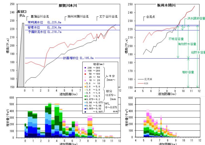
図-2.1.16 長安ロダム堆砂の粒径別の縦断分布（平成26年度末時点）
