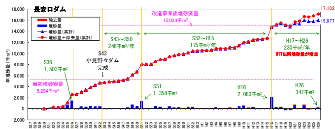
図-2.1.15 長安ロダムの堆砂量の経年変化
