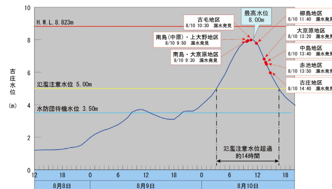
図-2.1.21 平成26年台風11号水位グラフ
