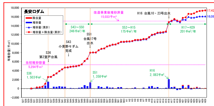
図-2.1.15 長安ロダムの堆砂量の経年変化
