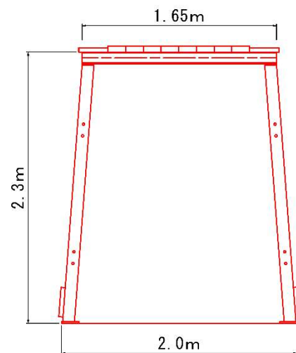
横坑正面図
