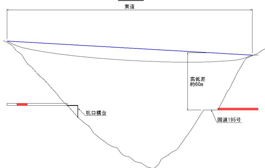
横断面図
