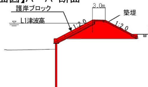
【断面図】A-A'断面
