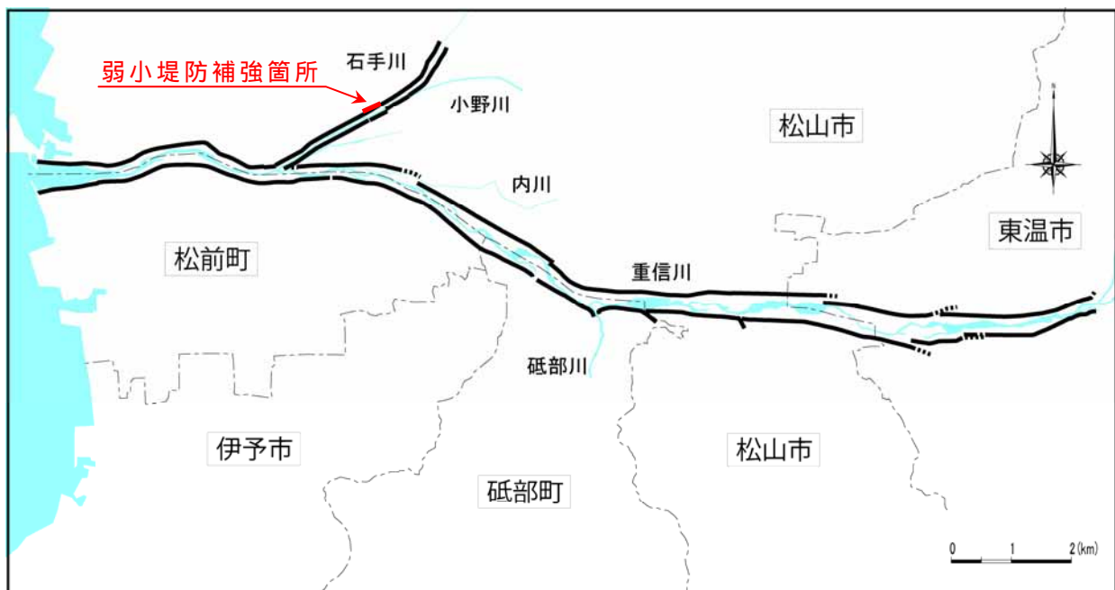
図-4.1.9 堤防補強区間位置箇所位置図を実施する箇所(石手川)
