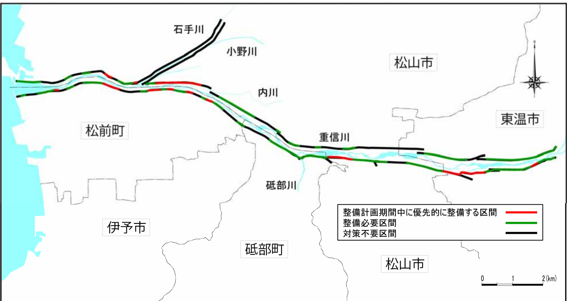
図-4.1.5 局所的な深堀れ対策を実施する区間
