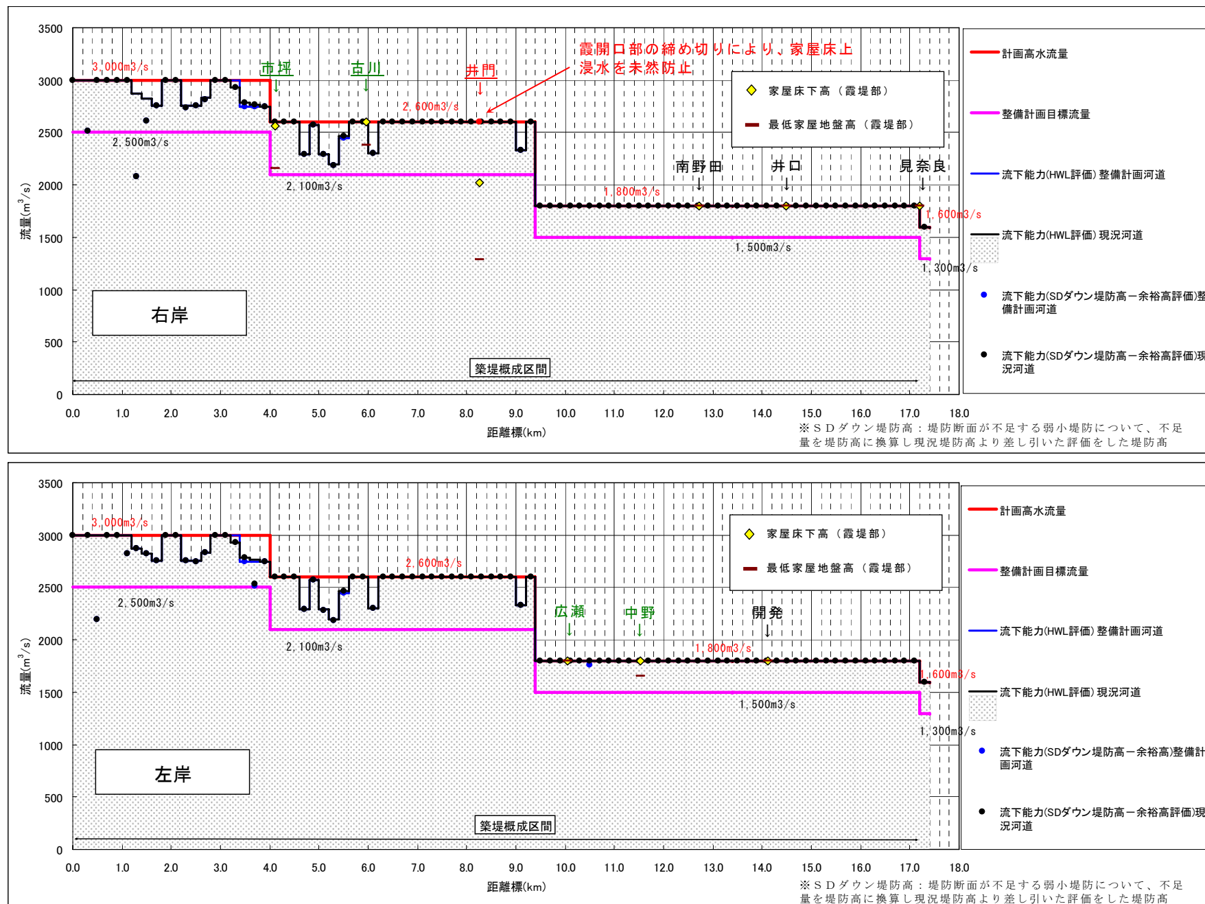
図-3.4.2 流下能力図【重信川】
