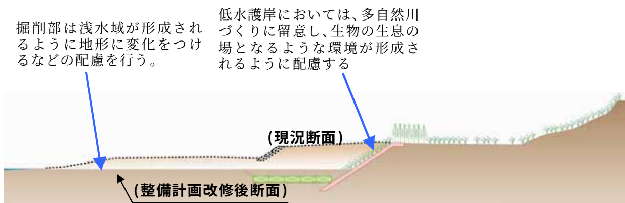
図-4.1.20 堤防の質的強化対策箇所の環境配慮イメージ（その1）
