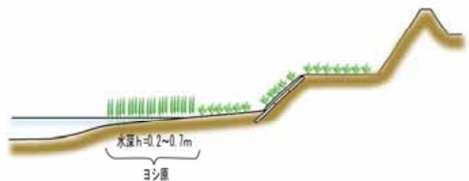
図-4.1.14 ヨシ原の再生の整備イメージ
