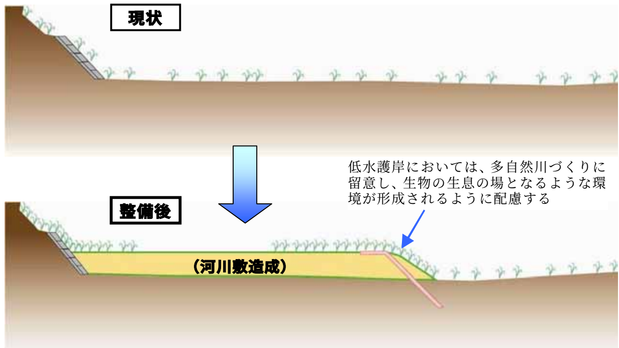
図-4.1.21 堤防の質的強化対策箇所の環境配慮イメージ（その2）
