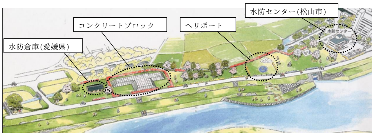
図-4.2.4 河川防災ステーション
