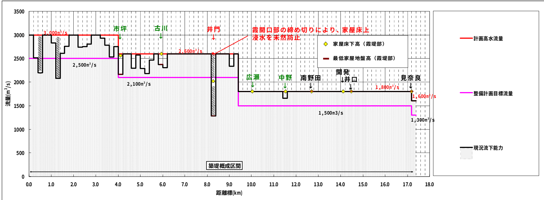
図-3.4.2 流下能力図【重信川】
