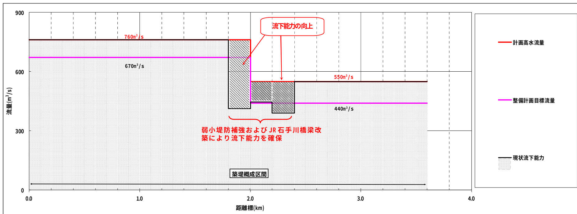
図-3.4.3 流下能力図【石手川】
