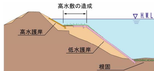
図-1.10局所洗掘・堤防侵食対策のイメージ図
