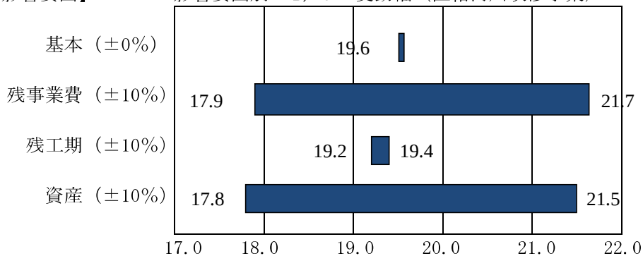
図-2.9 費用対効果の感度分析結果（残事業）
