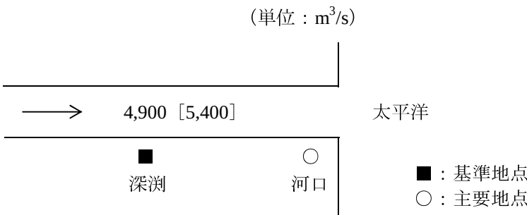
図-1.2 物部川水系計画高水流量配分図 ( [ ] は基本高水のピーク流量 )
