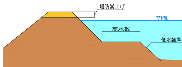
図-1.12堤防嵩上げのイメージ図
