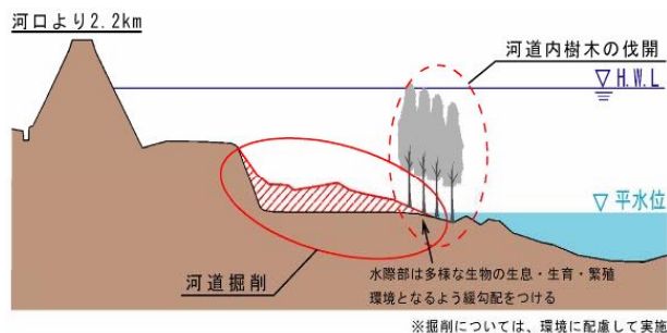
図-1.11河道掘削等のイメージ図
