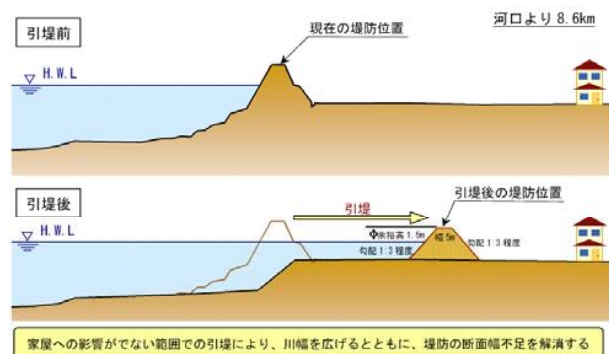
図-1.7 引堤イメージ
