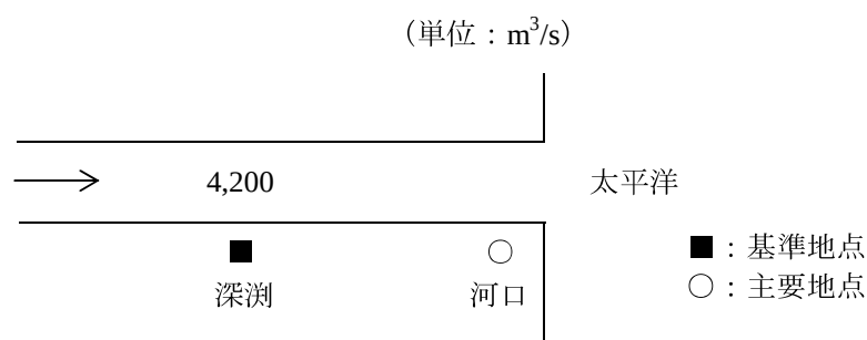
図-1.3 物部川河道目標流量配分図
