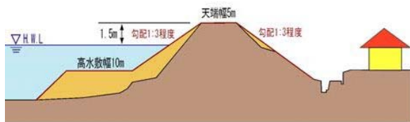
図-1.9堤防拡幅のイメージ図
