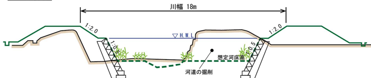
図4-5 長竹川の整備イメージ
