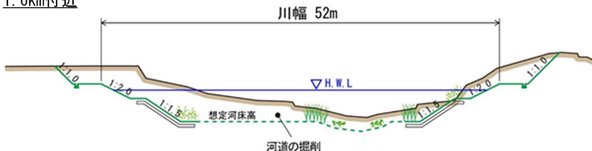
図4-3 日下川の整備イメージ
