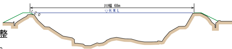
▲波介川 横断面図
