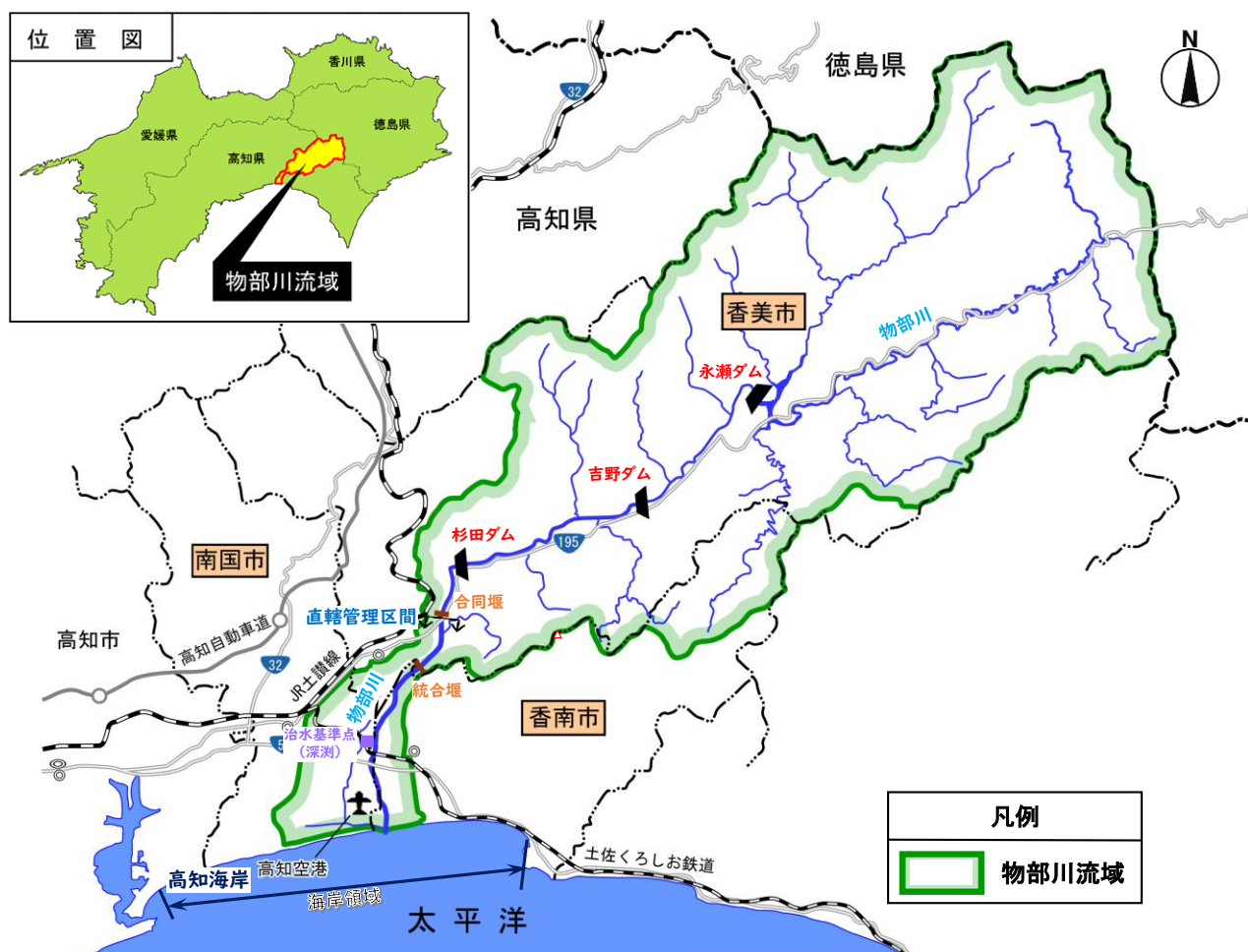
図-1 物部川流砂系の位置図
