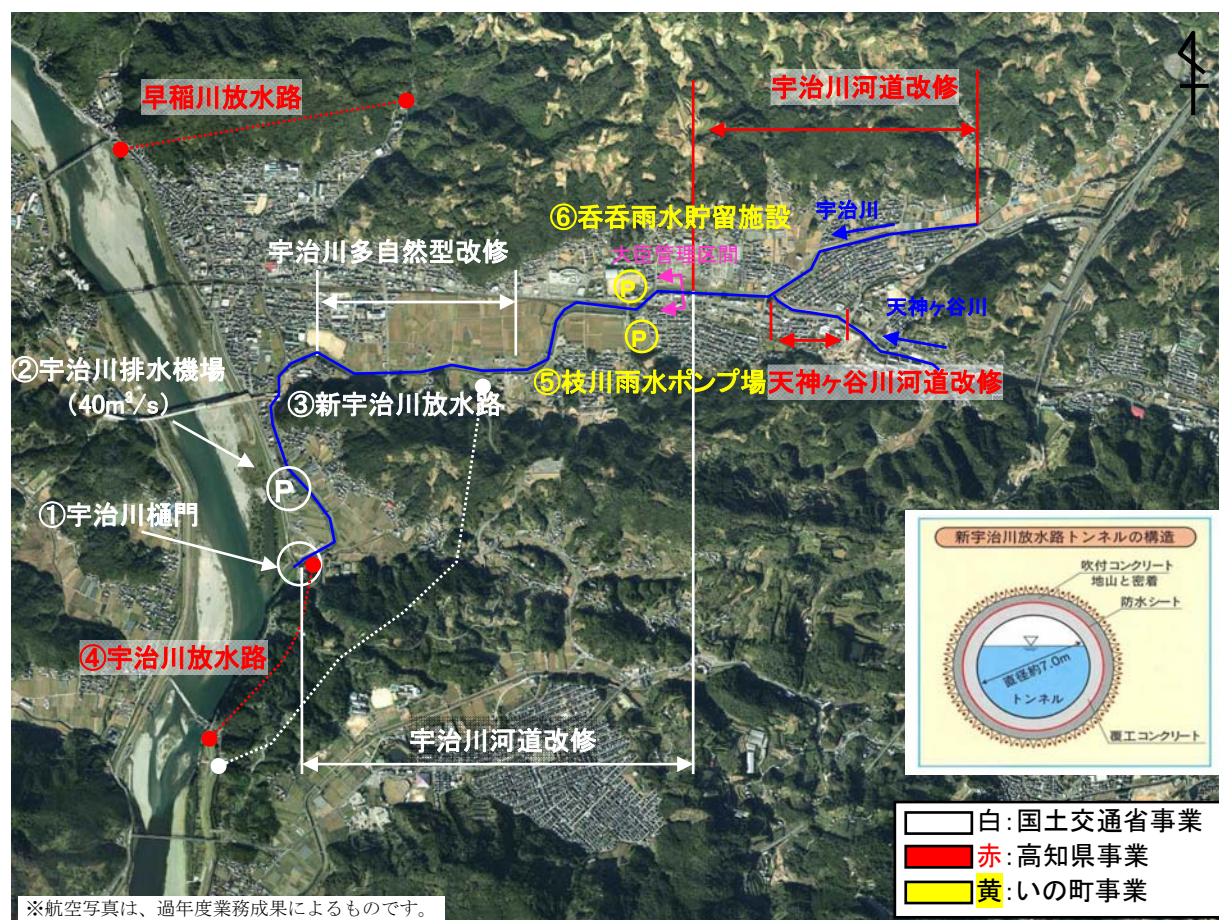
図 2.8 宇治川治水事業の位置図
