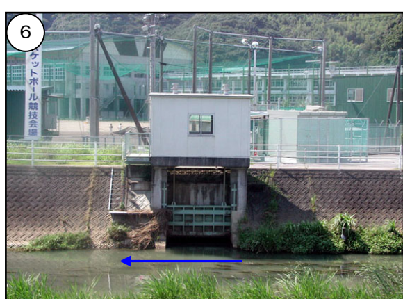
図 2.12 呑呑雨水貯留施設（呑呑樋門）
