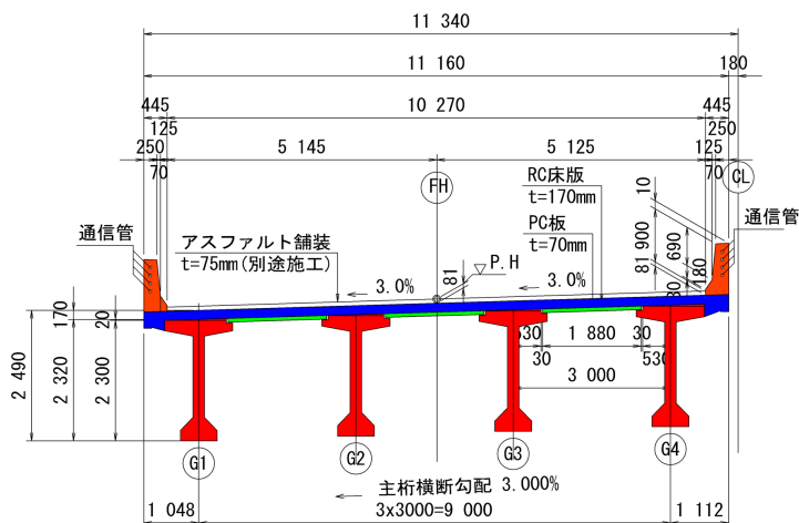
橋梁断面図
