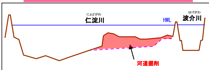
河道掘削の横断図イメージ
