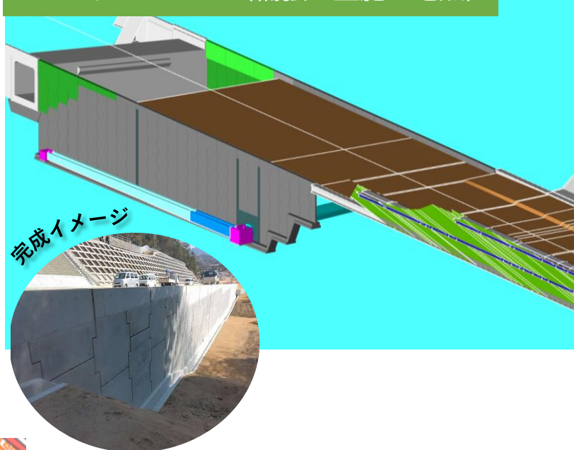
BIM/CIMデータ(補強土壁施工地点)
