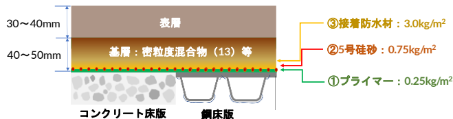
舗装断面のイメージ
