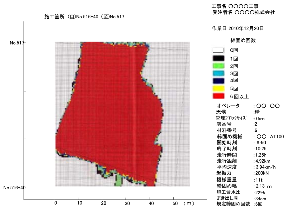
締固め回数分布図例（管理ブロックサイズ 0.50m）
