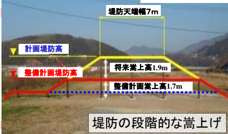
暫々定堤防嵩上げイメージ ..... 一部嵩上げ (H30年度完成予定)
