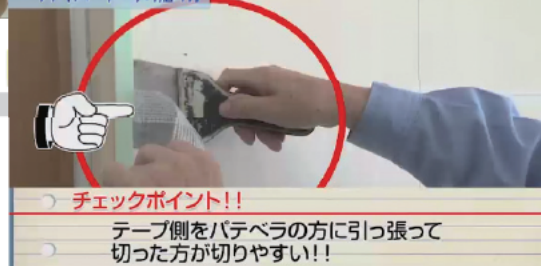
ファイバーテープの貼り方
