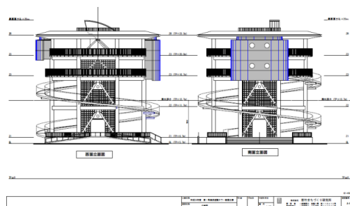
立面図（出典：中土佐町提供資料）
