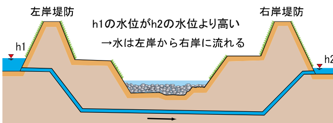
サイホンの概要図
