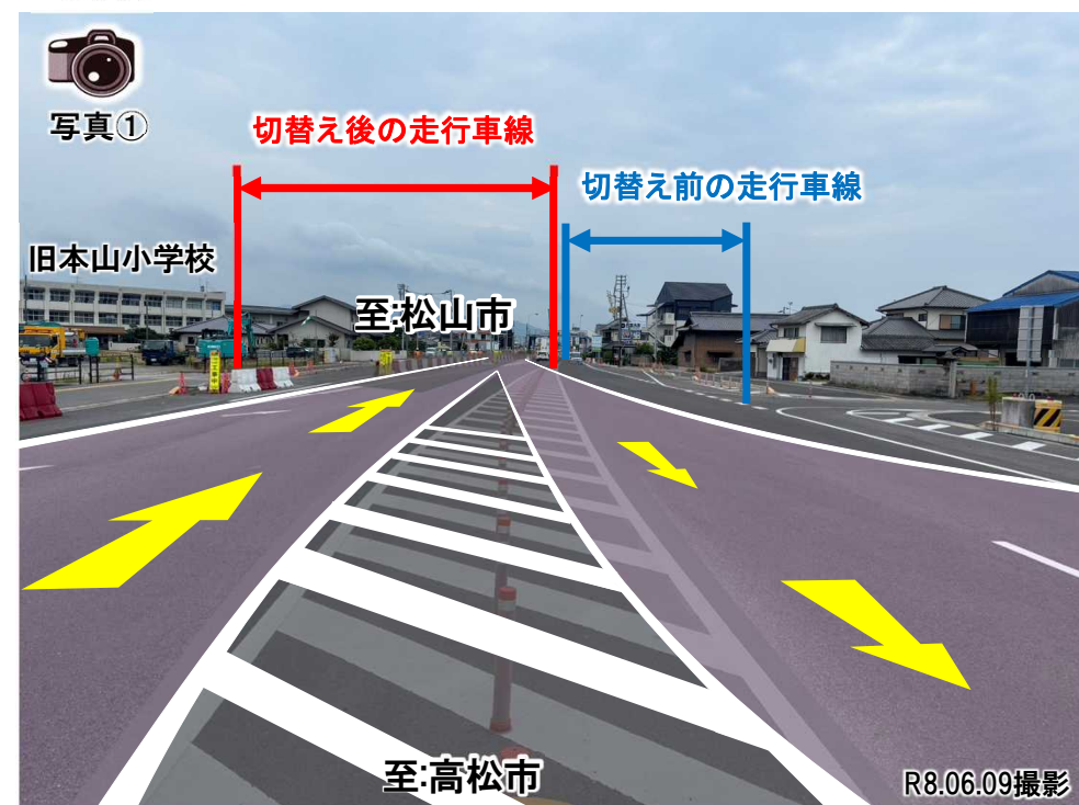
○高松側切り替え開始地点より松山方面を望む(写真①)
